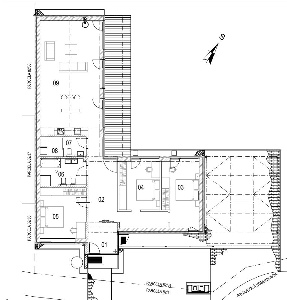
PÔDORYS 1.NP, M=1:200
