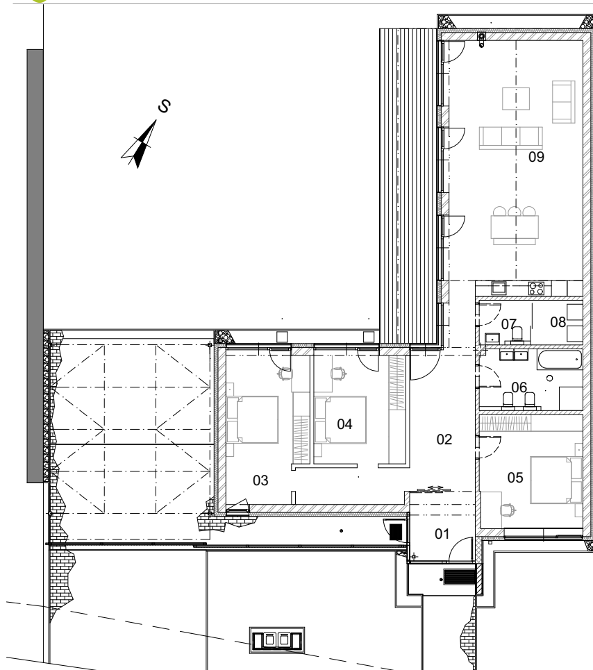
PÔDORYS 1.NP, M=1:200
