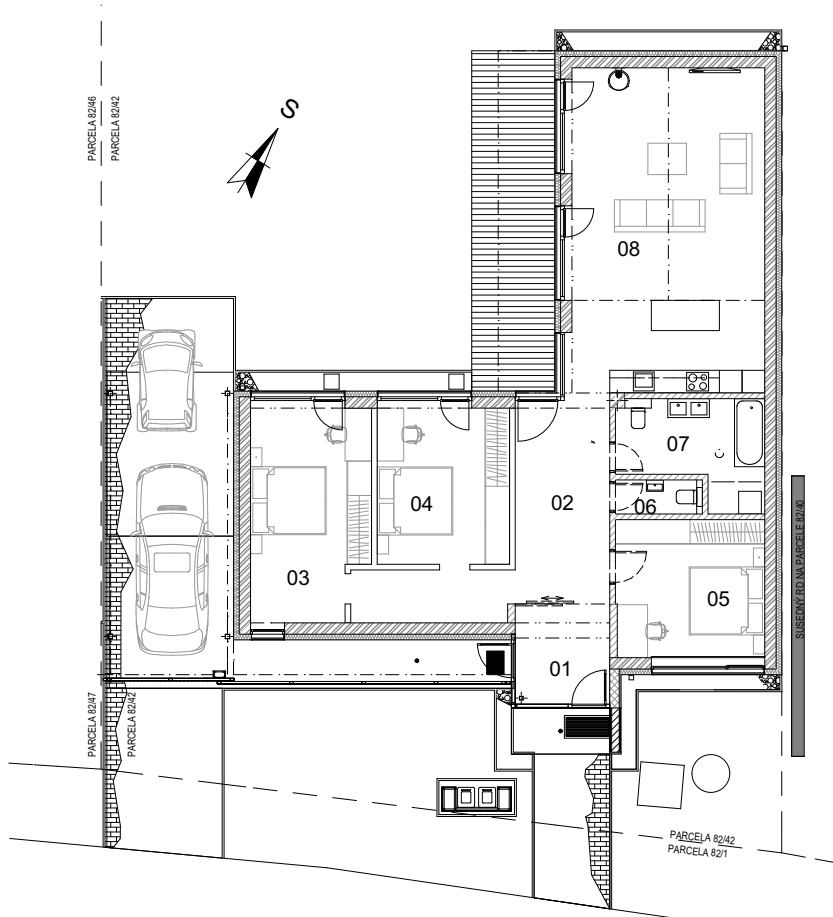
PÔDORYS 1.NP, M=1:200
