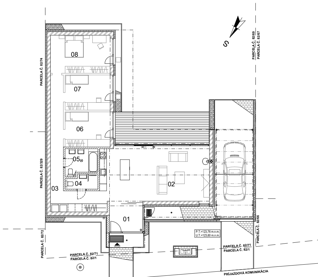
PÔDORYS 1.NP, M=1:200
