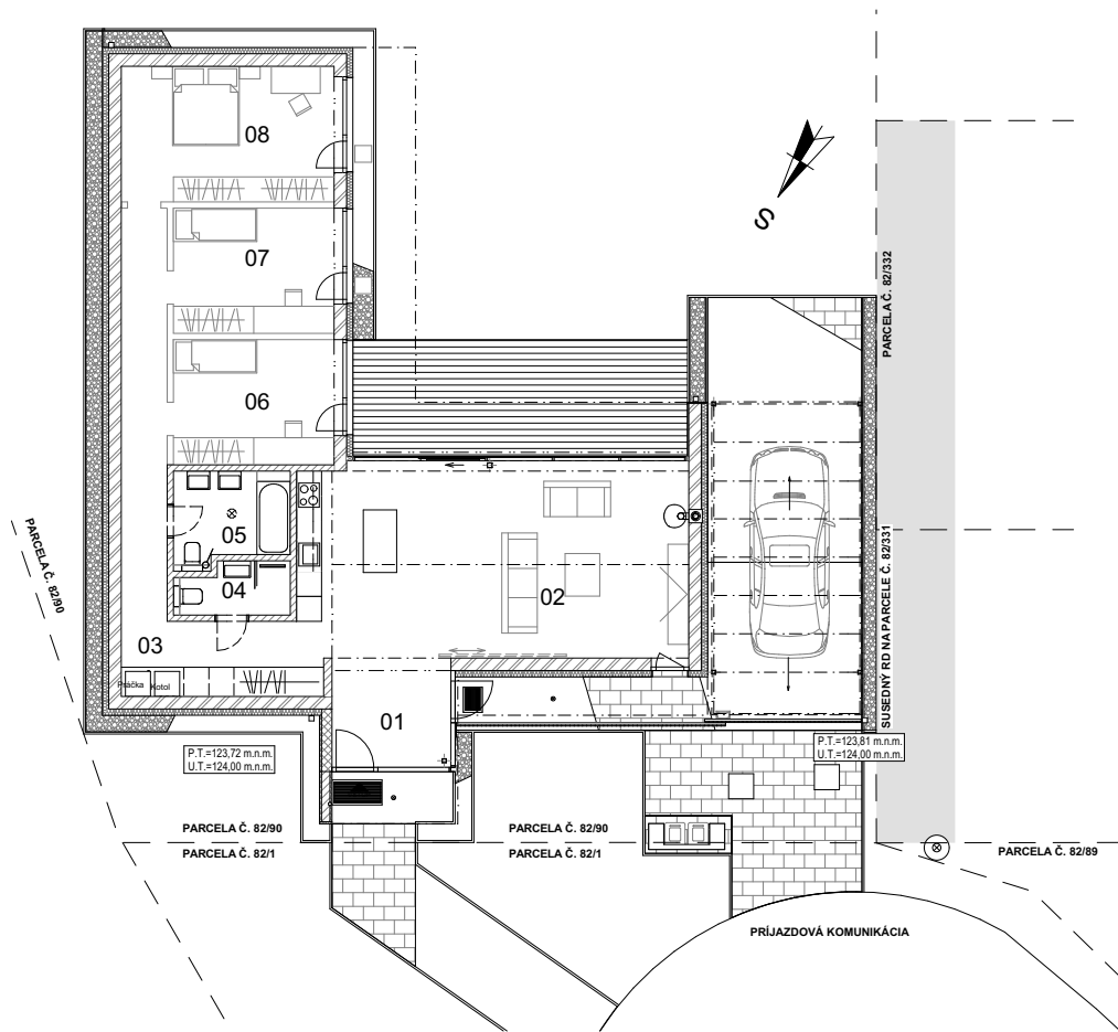
PÔDORYS 1.NP, M=1:200
