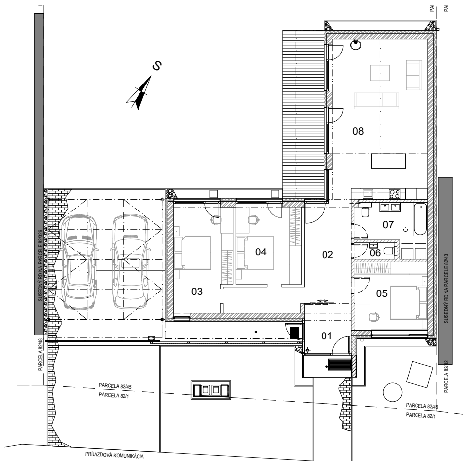
PÔDORYS 1.NP, M=1:200
