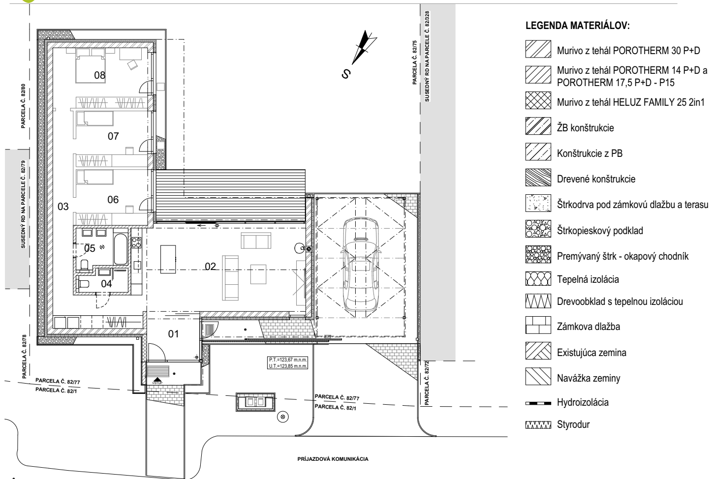
PÔDORYS 1.NP, M=1:200
